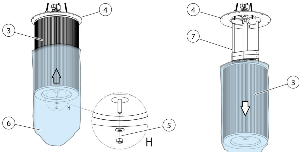
Abb. 68: Filterwechsel – Filterpatrone demontieren
