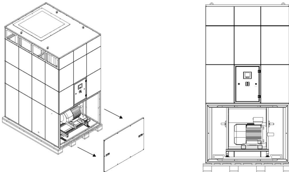
Abb. 9: Ventilatoreil Wartungstür öffnen
