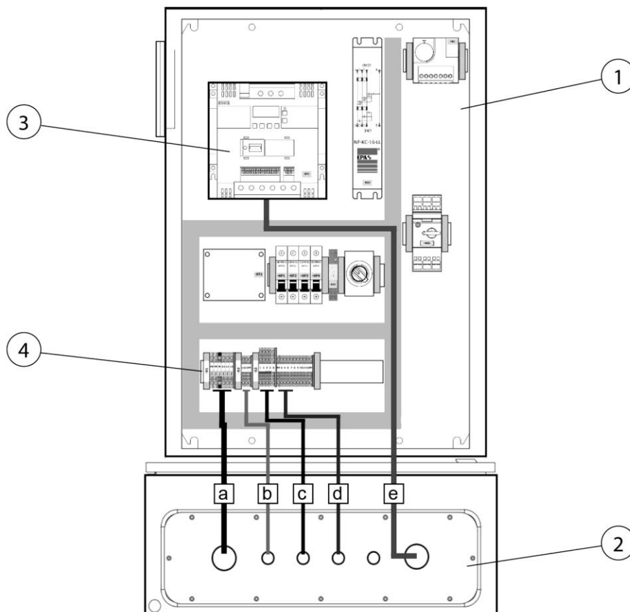
Abb. 34: Schaltschrank Absaugleistungsregelung
