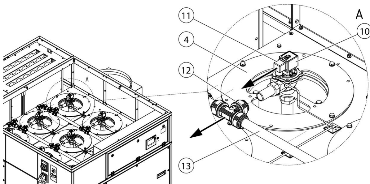
Abb. 65: Filterwechsel – Anschlüsse demontieren
