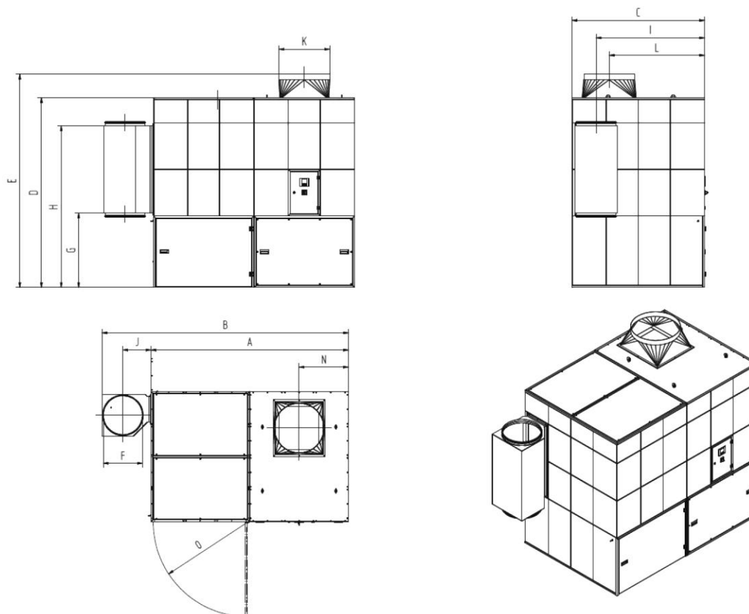
Abb. 76: Maßblatt 34130
