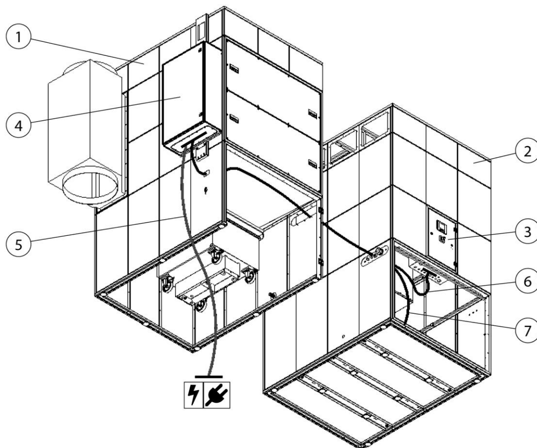
Abb. 33: Beispiel: Kabelverlegung Absaugleistungsregelung
