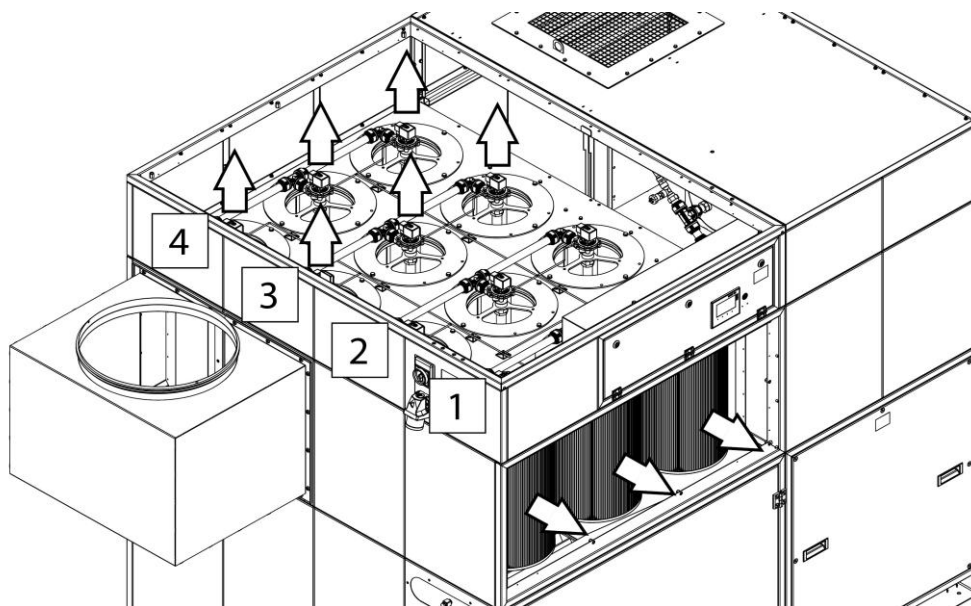
Abb. 61: Filterwechsel
