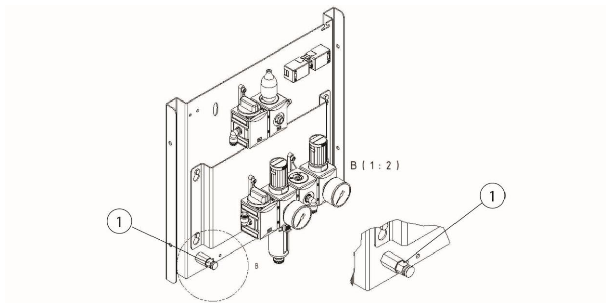
Abb. 70: Kondensatablassventil Druckluftbehälter
