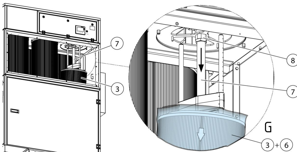
Abb. 63: Rotationsdüse demontieren
