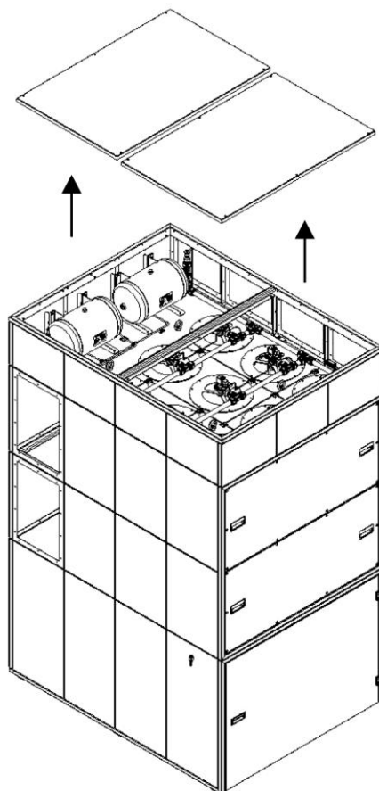
Abb. 17: Abdeckbleche entfernen
