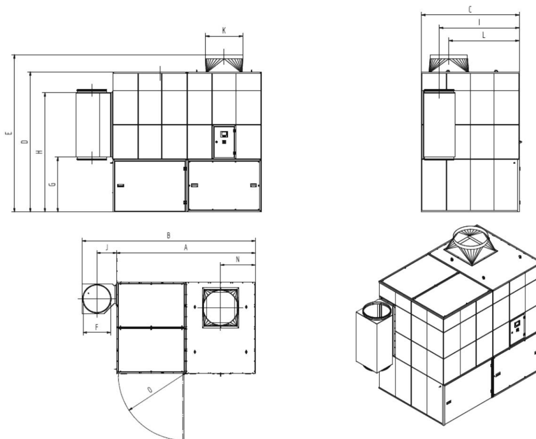
Abb. 75: Maßblatt 34110
