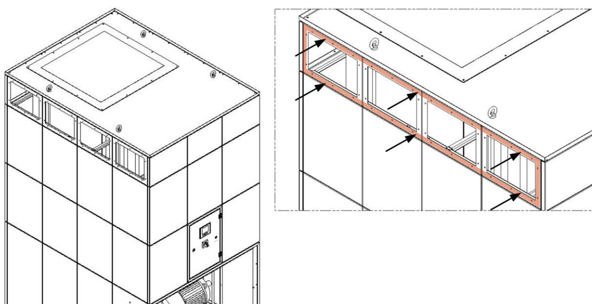
Abb. 12: Reinluftdurchgang
