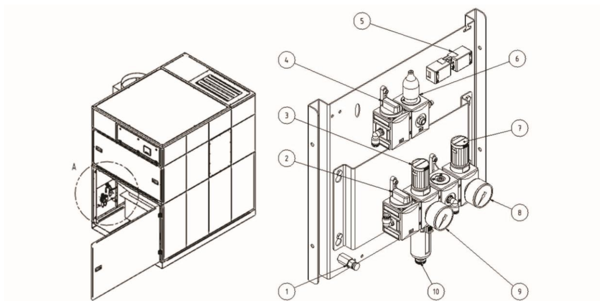
Abb. 27: Drucklufteinheit
