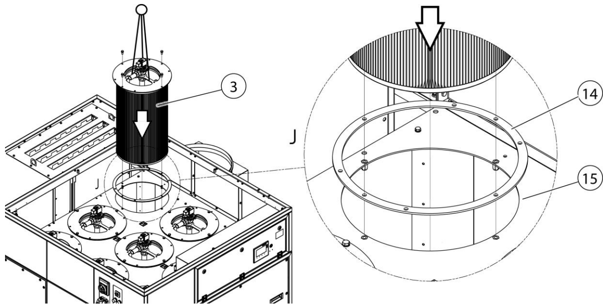
Abb. 69: Filterwechsel – Dichtung Filteraufnahme
