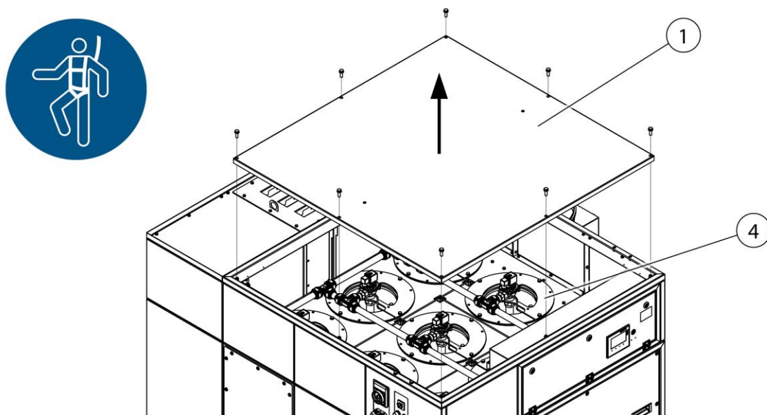
Abb. 64: Filterwechsel – Deckelblech demontieren
