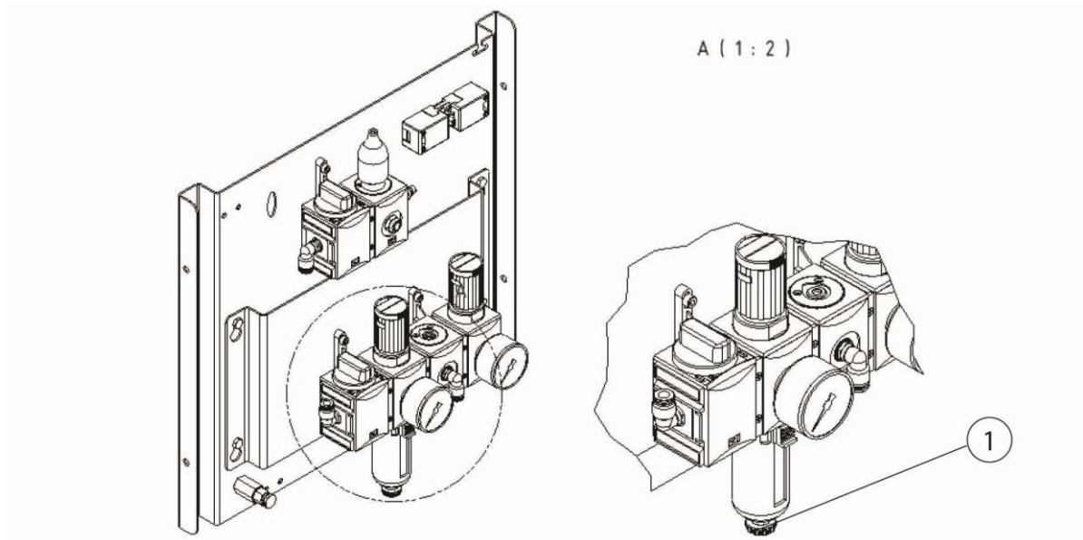
Abb. 71: Kondensatablassventil Druckluftwartungseinheit
