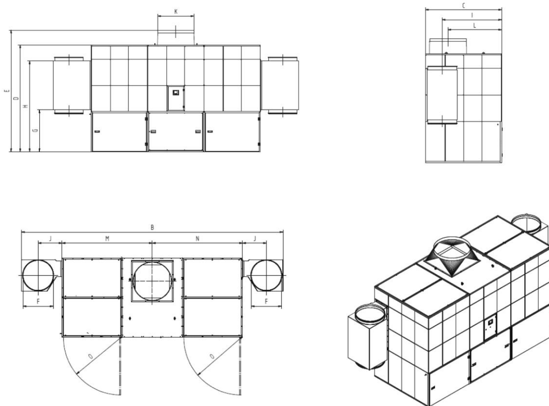
Abb. 78: Maßblatt 34180
