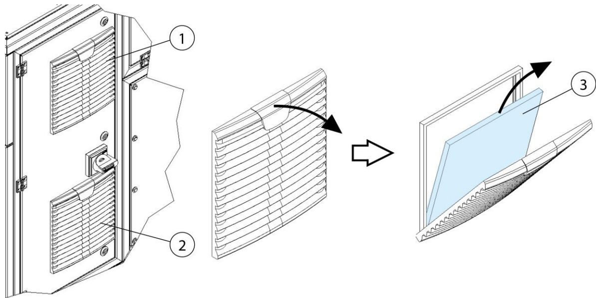
Abb. 57: Filterwechsel Schaltschrank-Entwärmung
