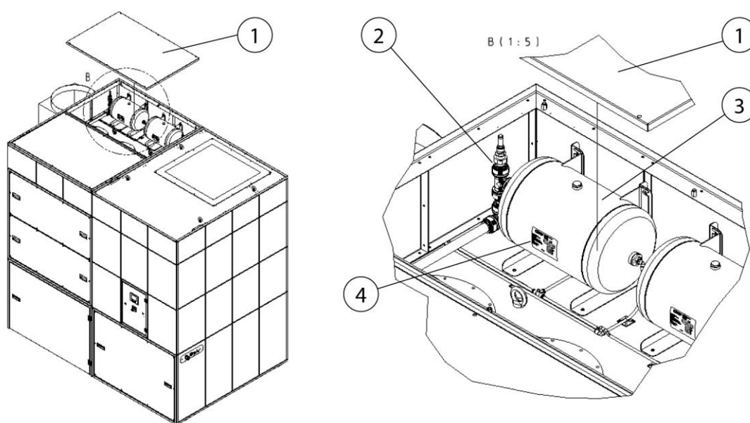
Abb. 74: Zugang zum Druckluftbehälter + Sicherheitsventil
