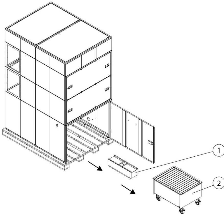
Abb. 16: Staubsaammelbehälter und Hebevorrichtung entfernen
