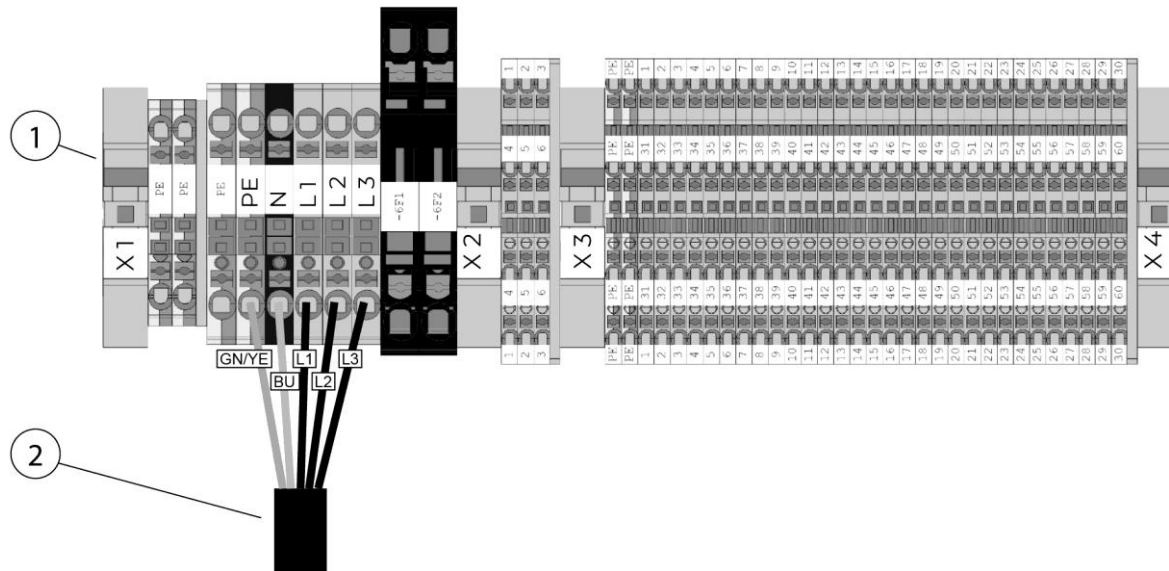
Abb. 32: Anschlussklemmenleiste Schaltschrank Produkt
