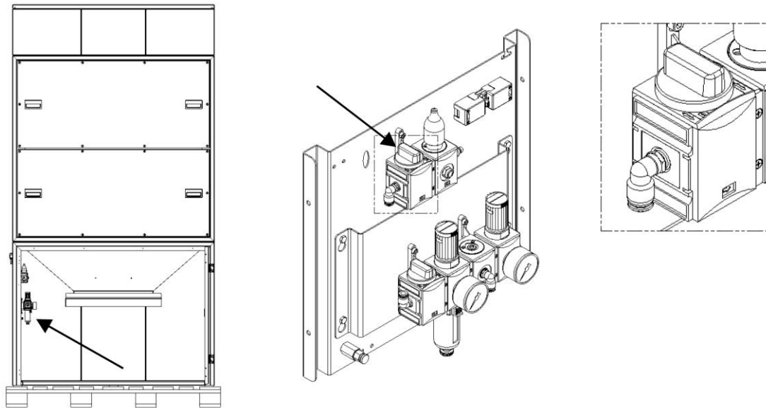
Abb. 14: Absenkventil Staubsammelbehälter
