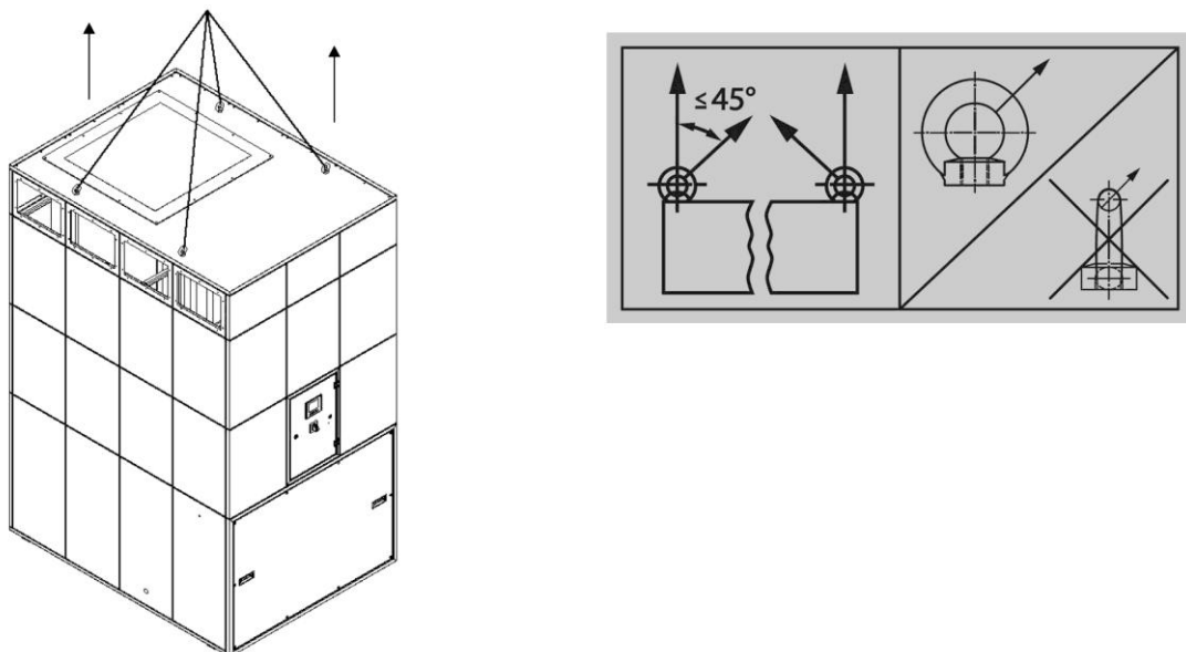
Abb. 10: Anheben Ventilatoreil mit Kran
