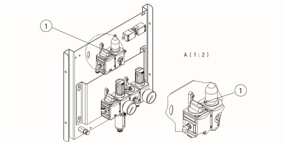
Abb. 55: Druckluftventil Staubsammelbehälter
