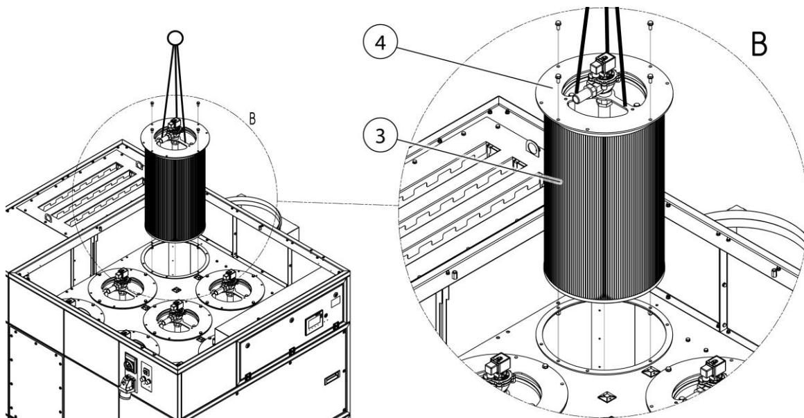
Abb. 67: Filterwechsel – Filteraufnahme demontieren
