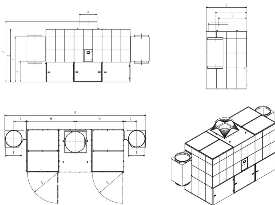
Abb. 77: Maßblatt 34160
