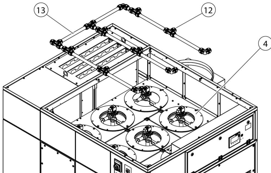
Abb. 66: Filterwechsel – Druckluftverrohrung demontieren
